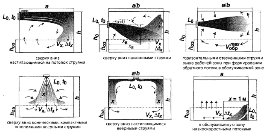
Рисунок Л.1 - Основные схемы подачи приточного воздуха
